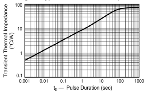
Fig. 8 – Typ. Transient Thermal Impedance
